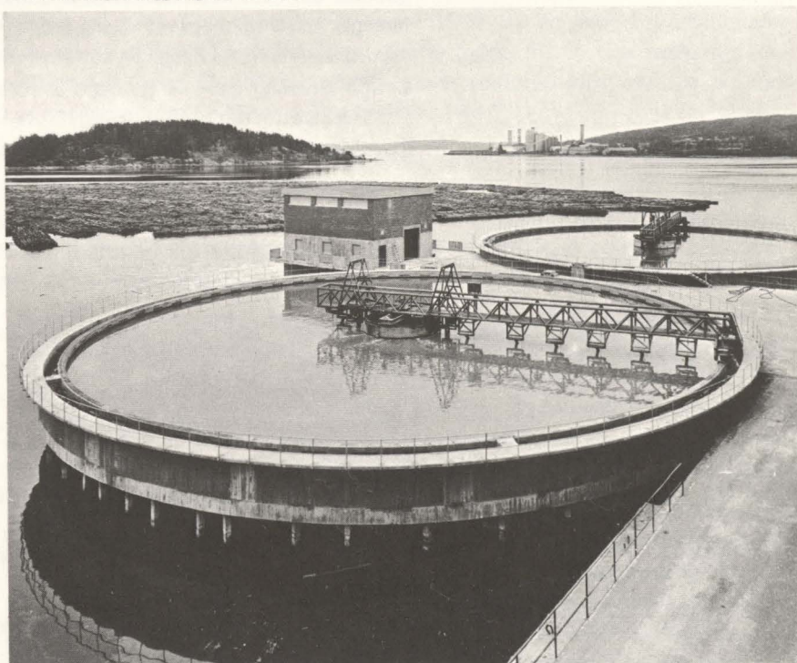
Sedimenteringsanläggning vid Ortviken
