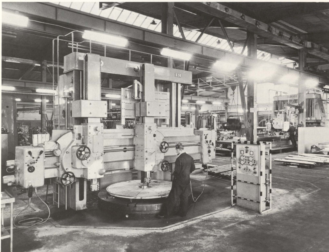
Bearbetning av tunga detaljer till cellulosa-maskiner vid Sundsbruk
