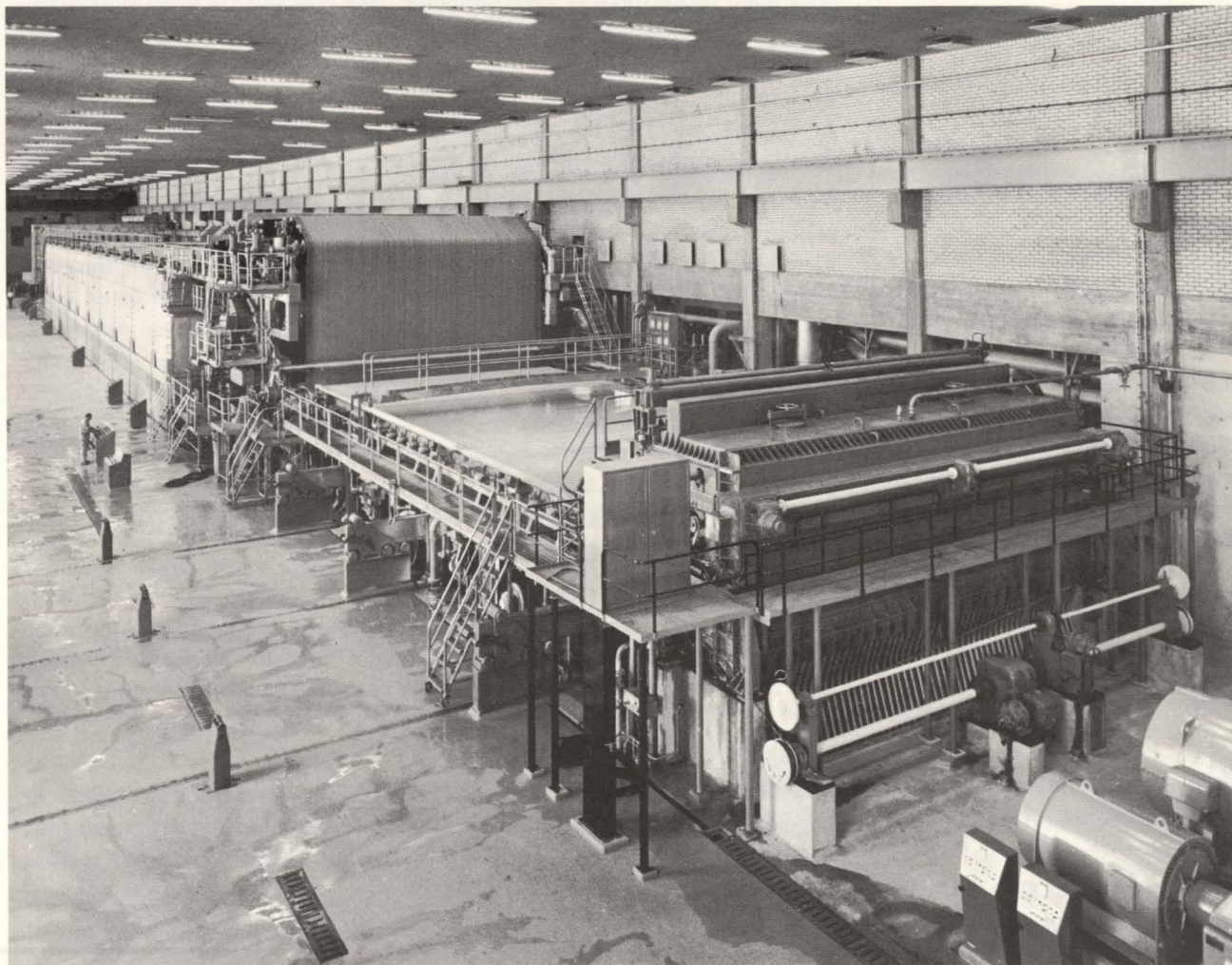
Den nya tidningspappersmaskinen i Ortviken
