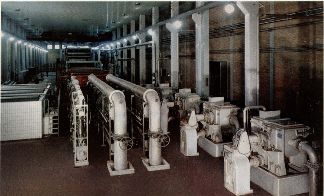
Anläggning för silning och virvelrening av blekt cellulosa (Nymölla AB, Nymölla).
