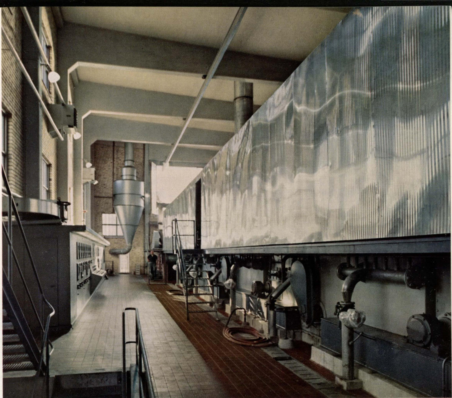
Anläggning för kontinuerlig tvättning och svartlutåtervinning på filter enligt system SUND-IMPCO (AB Statens Skogsindustrier, Karlsborgs Bruk).
