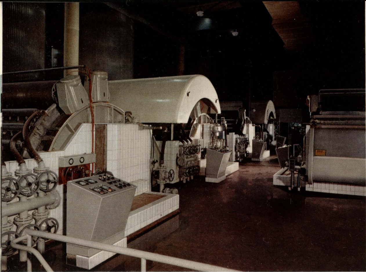
Anläggning för kontinuerlig blekning av magnesiumbisulfitcellulosa (Nymölla AB, Nymölla).
