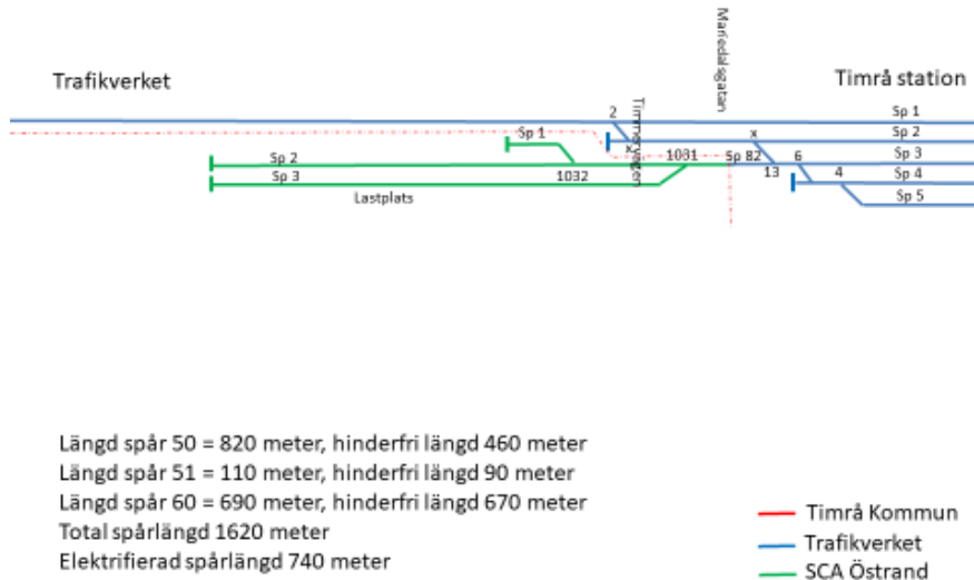
Bild 1. Järnvägsanläggning spår och spårväxlar SCA Östrand
